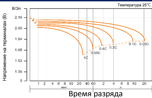
Кривые разряда
